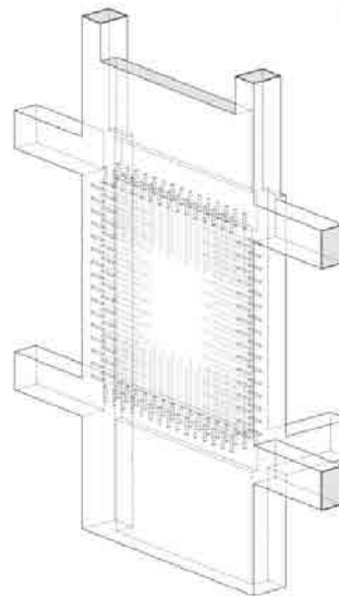
PARTICOLARE TIPOLOGICO DEGLI INTERVENTI DI CONSOLIDAMENTO DEI TELAI
